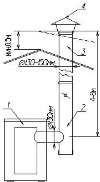
Рис. 1 Схема установки дымовой трубы
